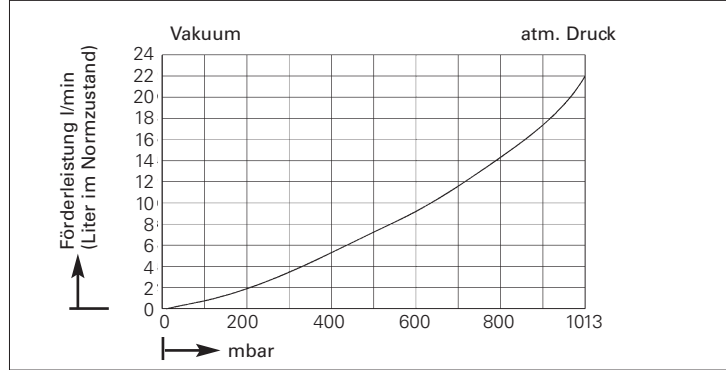
Leistungskurve
