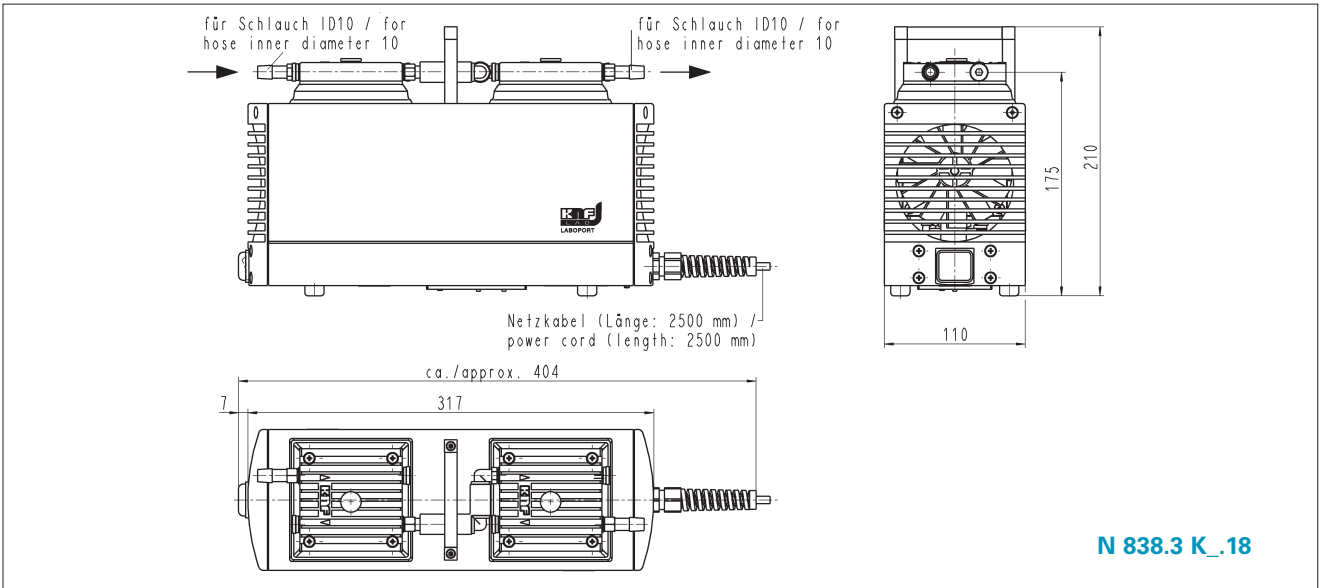
Maße (mm)
